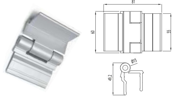
M05-502 ALDOKS GEÇME MENTEŞE HINGE
