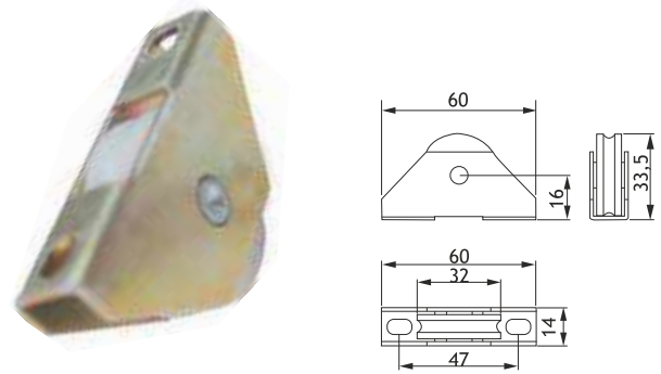
M10-516 METAL GÖVDE METAL ROLLER
