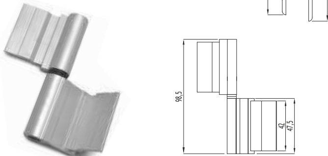
M05-501 ALDOKS MENTEŞE ALDOKS HINGE
