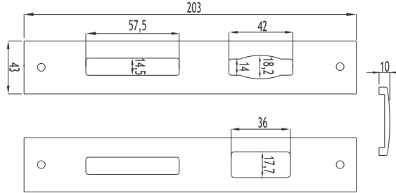
M06-504 C-60 KİLİT KARŞILIĞI C-60 STRIKER
