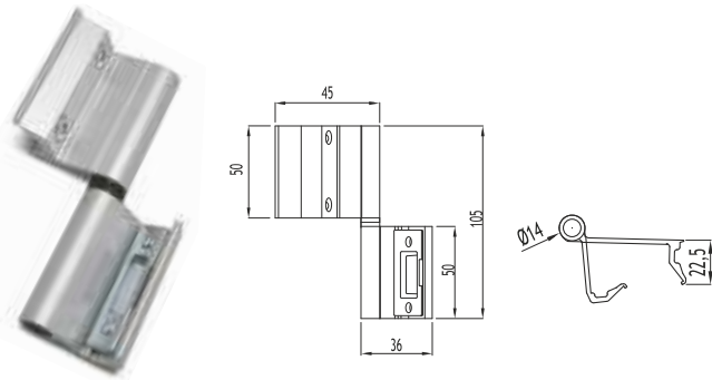
M05-503 SİSTEM PENCERE MENTEŞE SYSTEM WINDOW HINGE
