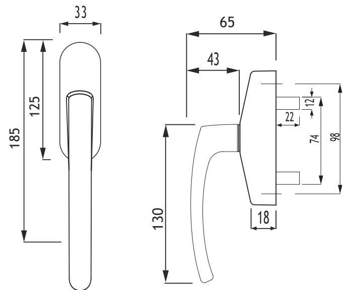
M01-502 MİESSO EKSENEL KOL ÇİFT DİLLİ MİESSO WINDOW HANDLE
