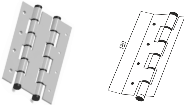
M05-505 YAYLI ÇARPMA KAPI MENTEŞESİ ( BAR MENTEŞE ) BAR DOOR HINGE
