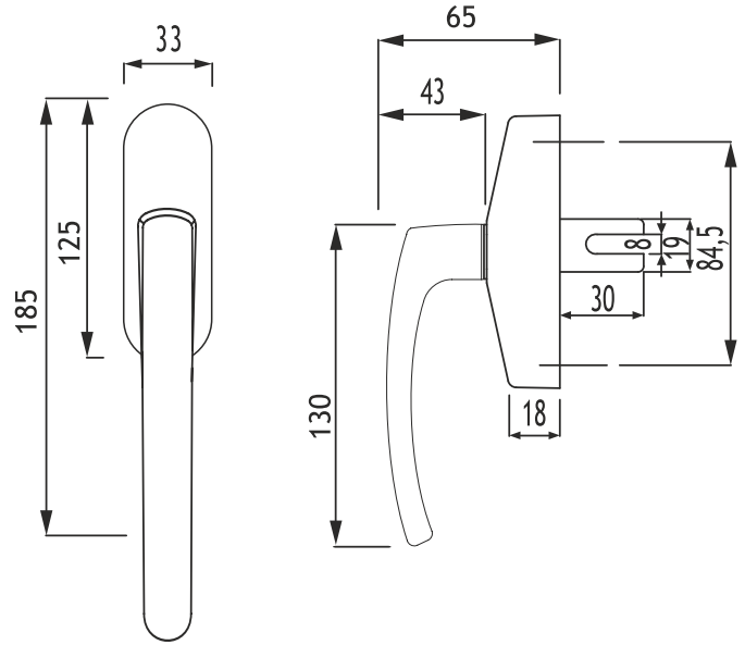
M01-501 MİESSO EKSENEL KOL TEK DİLLİ MİESSO WINDOW HANDLE
