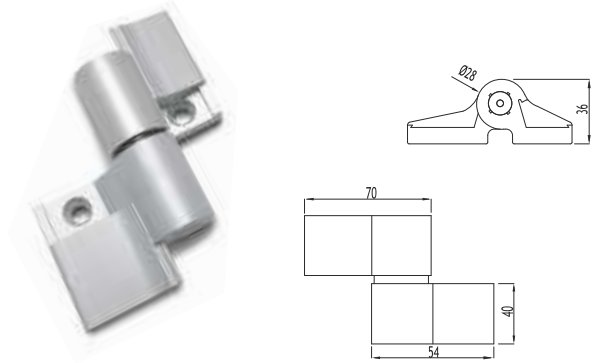
M05-504 KAPAZLAMA MENTEŞE HINGE
